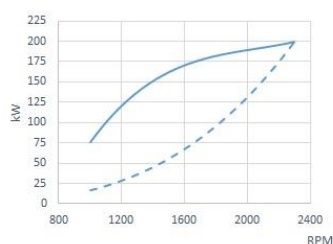
Effektkurva (ISO 3046/1)
