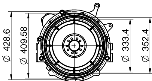
VISTA A
