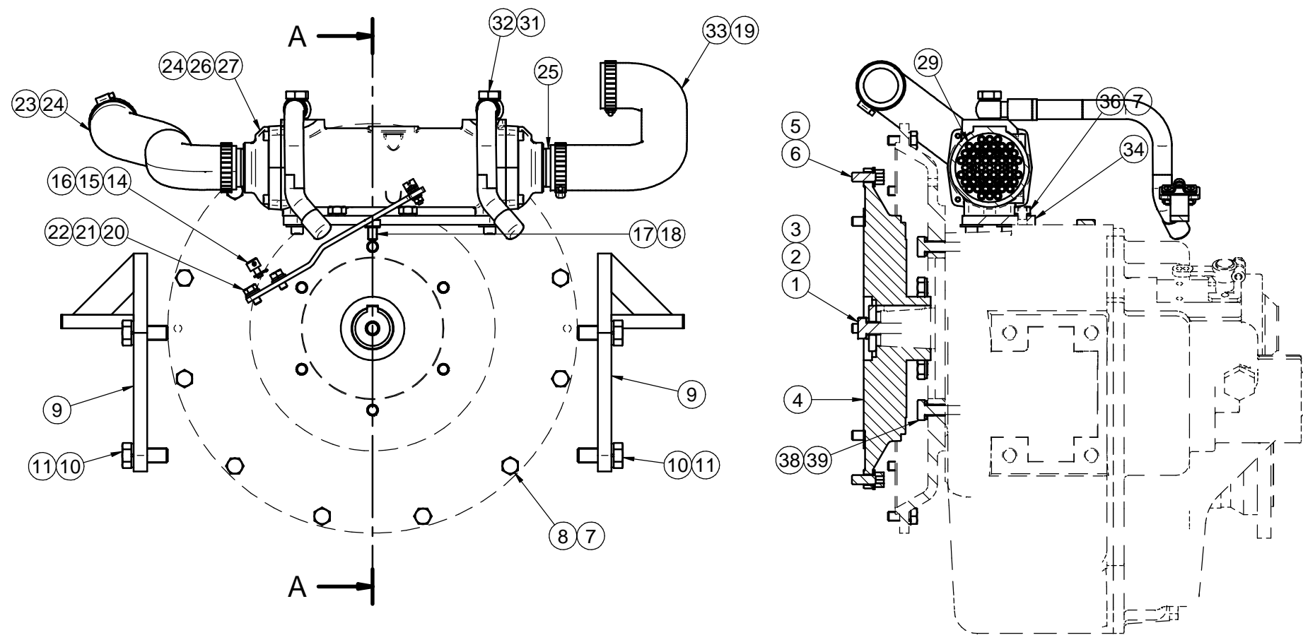
CORTE A-A
