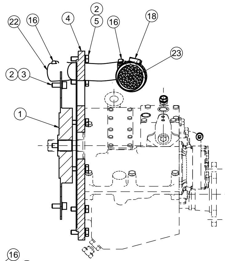
CORTE A-A
