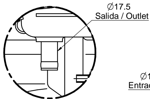
DETALLE A
