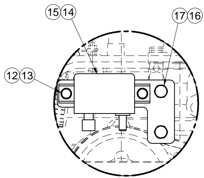
DETALLE A
