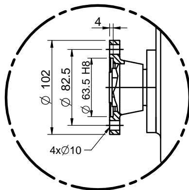
DETALLE A
