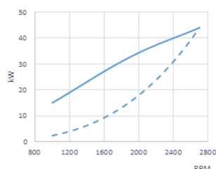
Effektkurva (ISO 3046/1)
