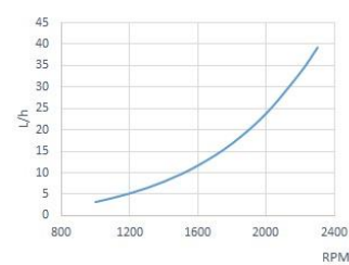
Potrošnja goriva
