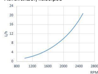
Κατανάλωση καυσίμου
