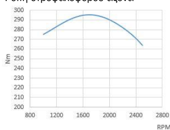
Ροπή στροφαλοφόρου άξονα
