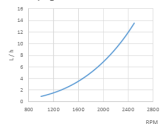
Potrošnja goriva
