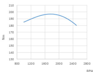
okretni moment na radilici
