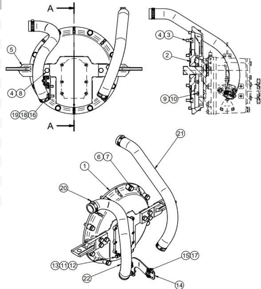
CORTE A-A
